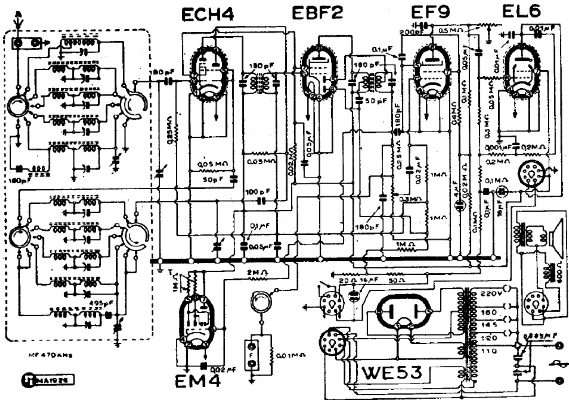
MINERVA - MOD. « 465/1 »
